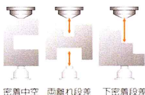
段差形態
